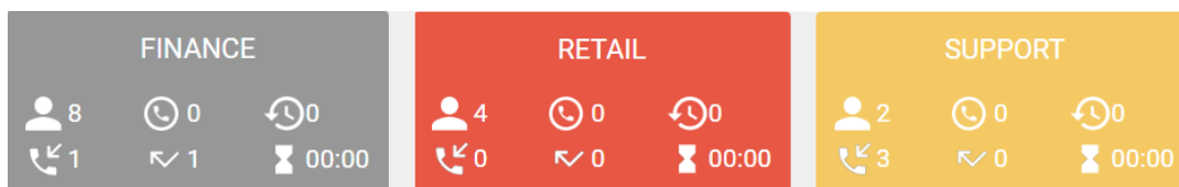
Afbeelding 3 Kleuren wachtrijen
